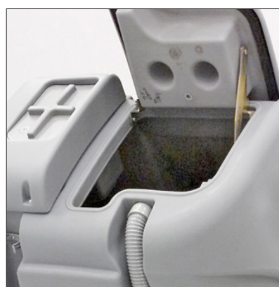
3. Prüfen/Reinigen des Sauggebläse-Schaumfilters (innen unter der Klappe Abb.).
