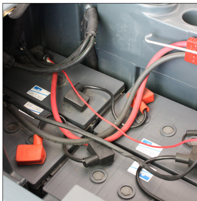
2. Batteriekontrolle – Füllstand der Säure überprüfen (bei Naßbatterien).
